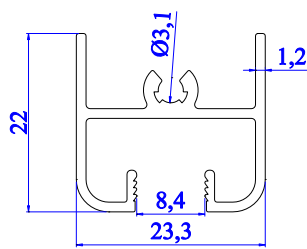
5154 - 0.248 kg/m
