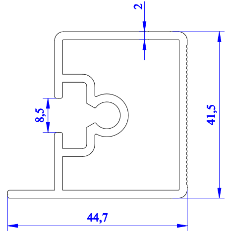
5264 - 1,010 kg/m
