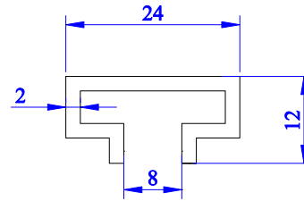
1761 - 0.304 kg/m
