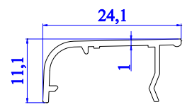
5185 - 0.117 kg/m
