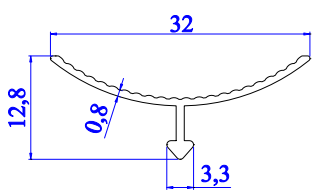
4858 - 0.110 kg/m
