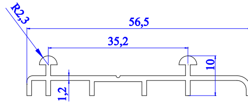
3999 - 0.322 kg/m
