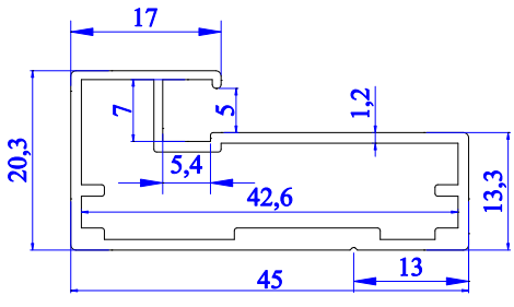
4710 - 0.518 kg/m
