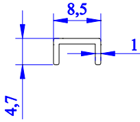
4127 - 0.043 kg/m
