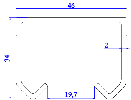
3888 - 0.700 kg/m
