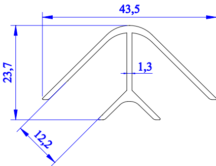
4031 - 0.338 kg/m
