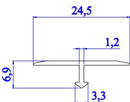
4650 - 0.090 kg/m
