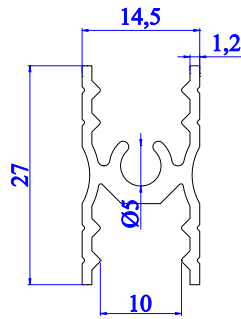
4715 - 0.313 kg/m
