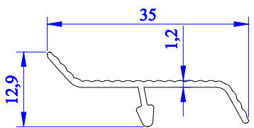
5387 - 0.152 kg/m
