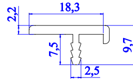
4970 - 0.163 kg/m
