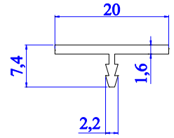
3935 - 0.109 kg/m
