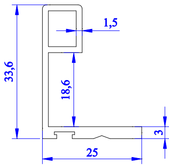
4965 - 0.406 kg/m
