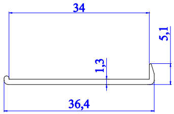
4847 - 0.139 kg/m
