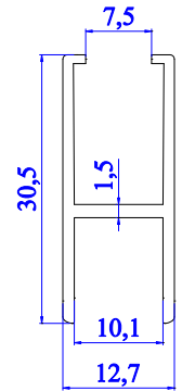
4813 - 0.255 kg/m
