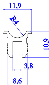
4734 - 0.137 kg/m
