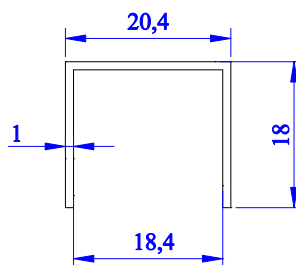
4289 - 0.147 kg/m
