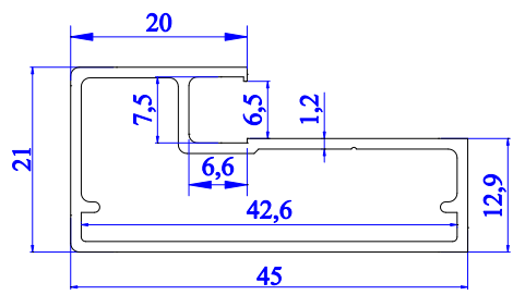
4933 - 0.449 kg/m
