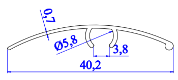
4017 - 0.121 kg/m
