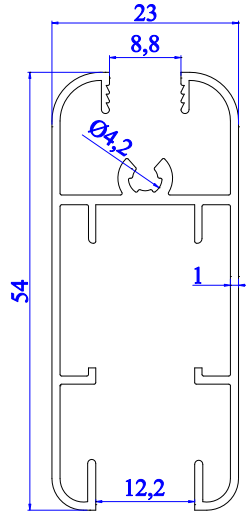
5156 - 0.535 kg/m
