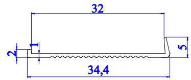
4927 - 0.090 kg/m
