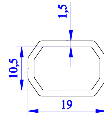
5166 - 0.211 kg/m
