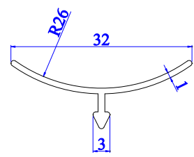
4857 - 0.119 kg/m
