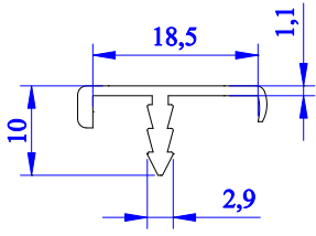
5341 - 0.134 kg/m
